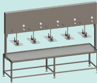
Gouda & Edam Cheese Press
